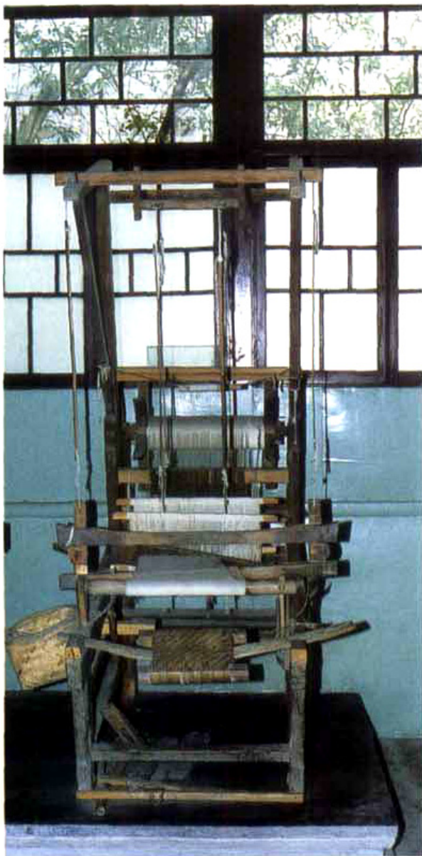
织布机
